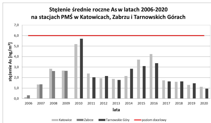
Rysunek 34. Stężenie średnie roczne arsenu na stacjach w Katowicach, Zabrze i Tarnowskich Górach (opracowanie własne na podstawie danych PM 10 )
