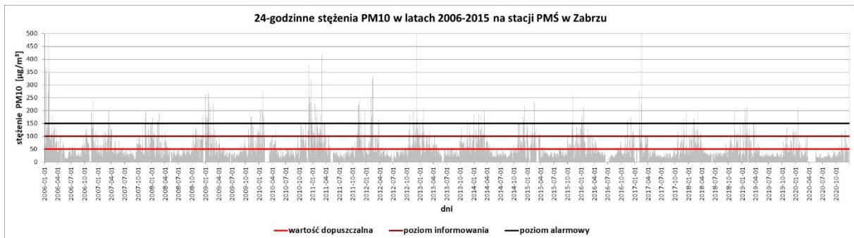
Rysunek 21. Stężenia 24-godzinne pyłu zawieszonego PM10 na stacji w Zabrzu (opracowanie własne na podstawie danych PMŚ)
