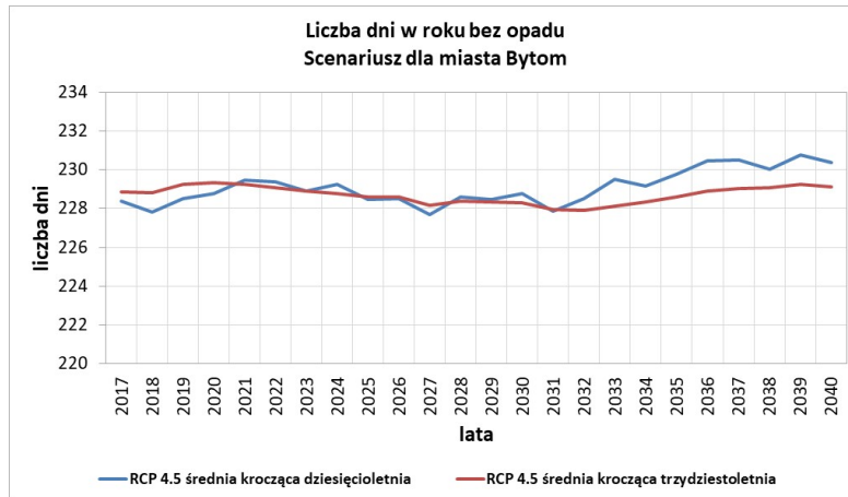
Rysunek 44. Liczba dni w roku bez opadu wg scenariusza RCP 4.5 dla miasta Bytom (opracowanie własne na podstawie projektu Klimada 2.0)
