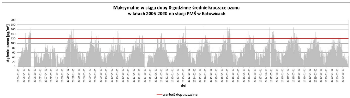
Rysunek 3. Stężenia maksymalne z 8-godzinnych średnich krocących w ciągu doby dla ozonu na stacji w Katowicach (opracowanie własne na podstawie danych PMS)
