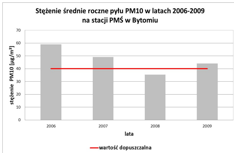
Rysunek 15. Stężenie średnie roczne pyłu zawieszzonego PM10 na stacji w Bytomiu (opracowanie własne na podstawie danych PMŚ)
