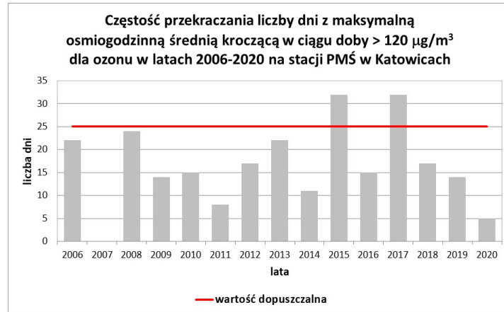
Rysunek 5. Częstość przekraczania docelowego stężenia ozonu ( 120 \mu\text{g}/\text{m}^3 , liczonego jako stężenie maksymalne z 8-godzinnych średnich krocących w ciągu doby) na stacji w Katowicach (opracowanie własne na podstawie danych PMŚ)
