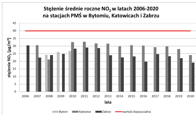
Rysunek 12. Stężenie średnie roczne dwutlenku azotu na stacjach w Bytomiu, Katowicach i Zabrze (opracowanie własne na podstawie danychch PMŚ)
