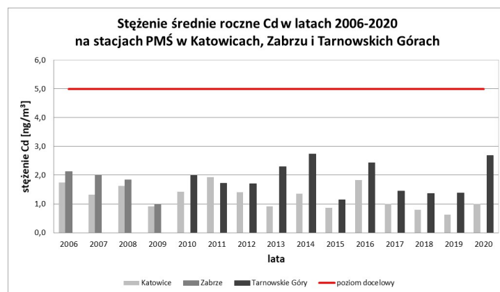
Rysunek 36. Stężenie średnie roczne kadmu na stacjach w Katowicach, Zabrze i Tarnowskich Górach (opracowanie własne na podstawie danych PMŚ)
