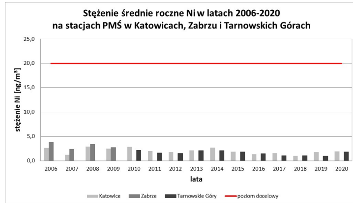
Rysunek 35. Stężenie średnie roczne niklu na stacjach w Katowicach, Zabrze i Tarnowskich Górach (opracowanie własne na podstawie danych PMŚ)
