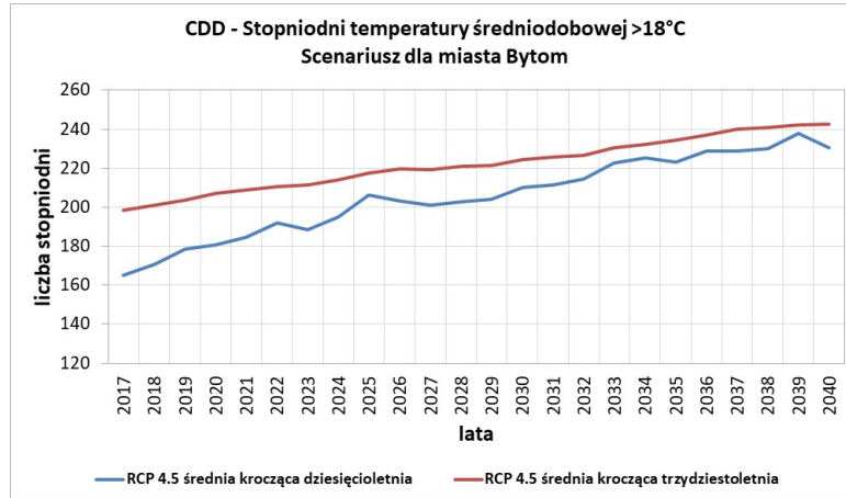
Rysunek 42. Liczba stopniocdni dla dni chłodzących, czyli z temperaturą średniodobową >18°C wg scenariusza RCP 4.5 dla miasta Bytom (opracowanie własne na podstawie projektu Klimada 2.0)
