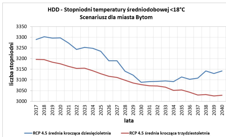
Rysunek 41. Liczba stopniodni dla dni grzewczych, czyli z temperaturą średniodobową <18°C wg scenariusza RCP 4.5 dla miasta Bytom (opracowanie własne na podstawie projektu Klimada 2.0)
