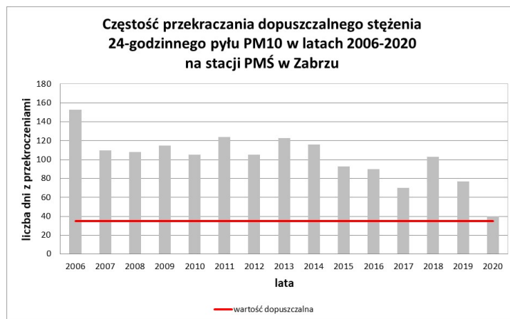
Rysunek 25. Częstość przekraczania dopuszczalnego stężenia 24-godzinnego pyłu PM10 na stacji w Zabrze (opracowanie własne na podstawie danych PMŚ)
