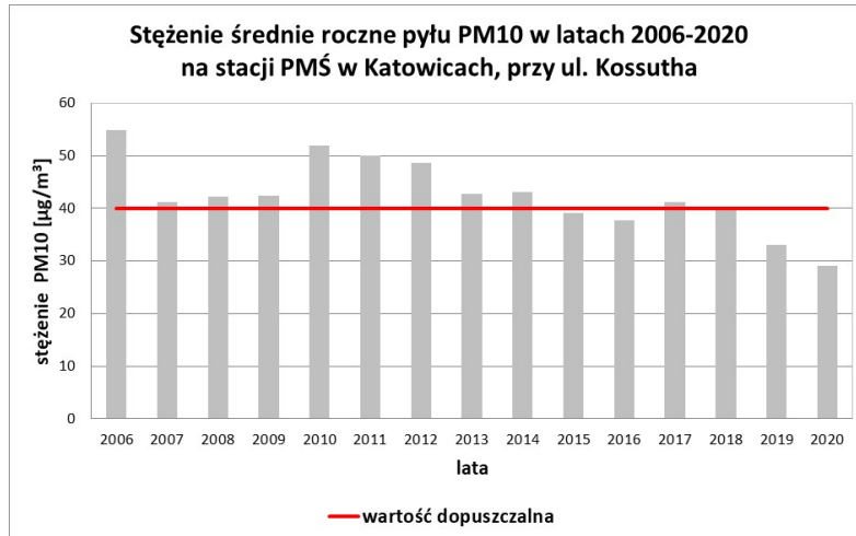
Rysunek 16. Stężenie średnie roczne pyłu zawieszonego PM10 na stacji w Katowicach (opracowanie własne na podstawie danych PMS)
