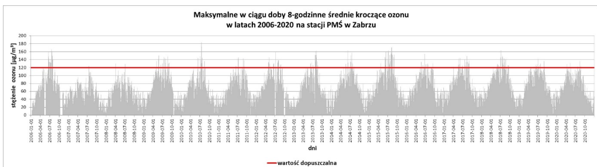
Rysunek 4. Stężenia maksymalne z 8-godzinnych średnich krocących w ciągu doby dla ozonu na stacji w Zabrzu (opracowanie własne na podstawie danych PMS)
