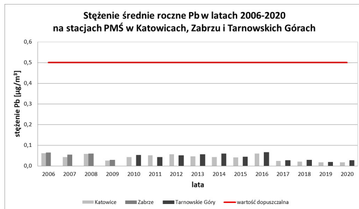
Rysunek 33. Stężenie średnie roczne ołowiu na stacjach w Katowicach, Zabrze i Tarnowskich Górach (opracowanie własne na podstawie danych PM 10 )
